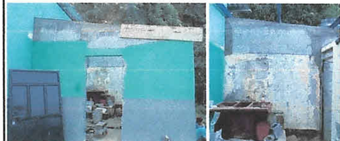
FOTO 6: RECONSTRUCCIÓN DE PARED, LEVANTADO DE ALTURA PARA EL CAMBIO DE PENDIENTE, COLOCACIÓN DE ESTRUCTURA Y LÁMINA.
